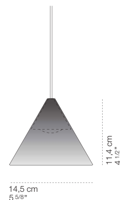
Cordina Conico Vetro Cromo-Tabacco
